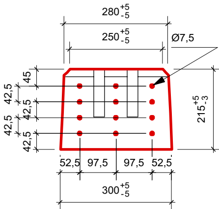
Coupe AA Ech: 1/10
