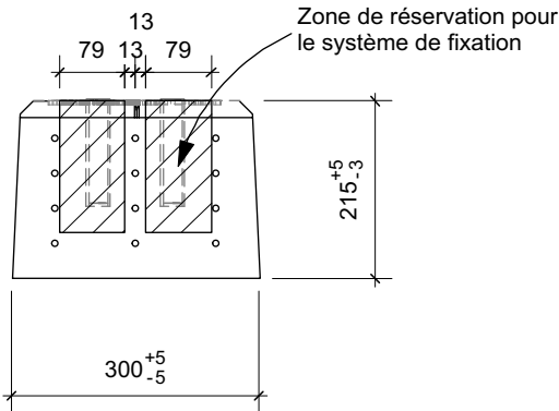
Vue de gauche Ech: 1/10
